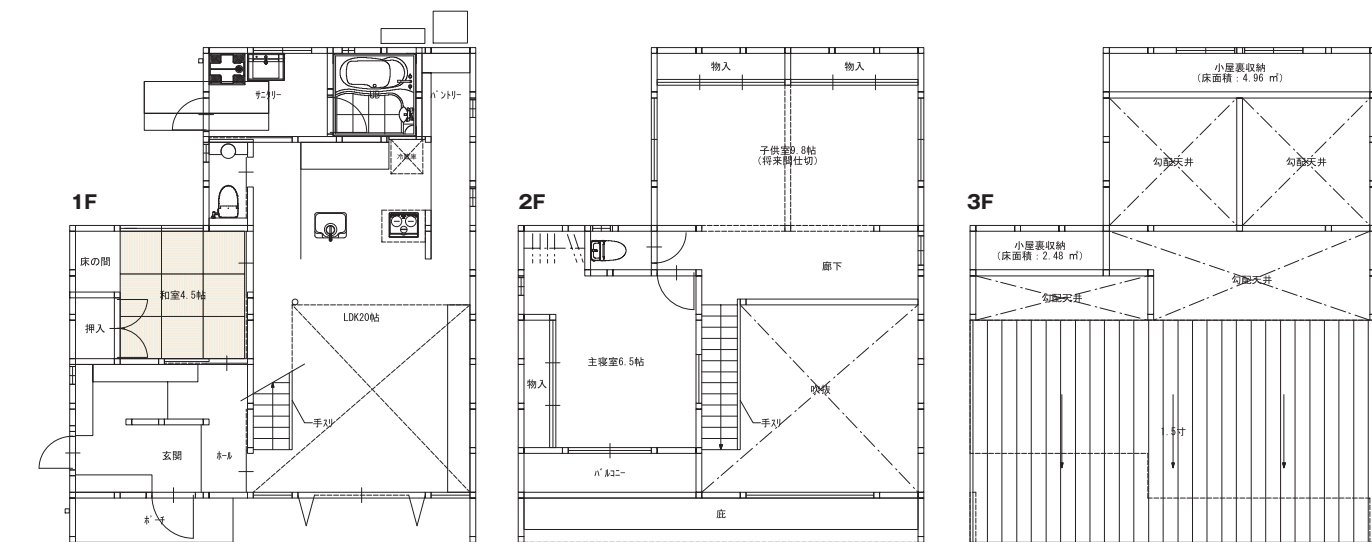
高知市 Y邸 DATA 設計・管理/株式会社 酒井建設 土地面積/331.53㎡(100.29坪) 延床面積/110.66㎡(33.47坪) 1F/64.59㎡(19.57坪) 2F/46.07㎡(13.93坪) 主な工法/木造在来工法 工期/4ヶ月
